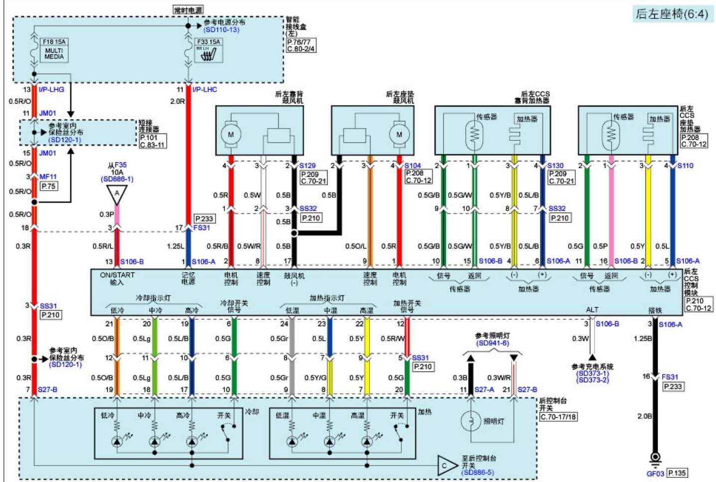
空调座椅控制系统(3)
